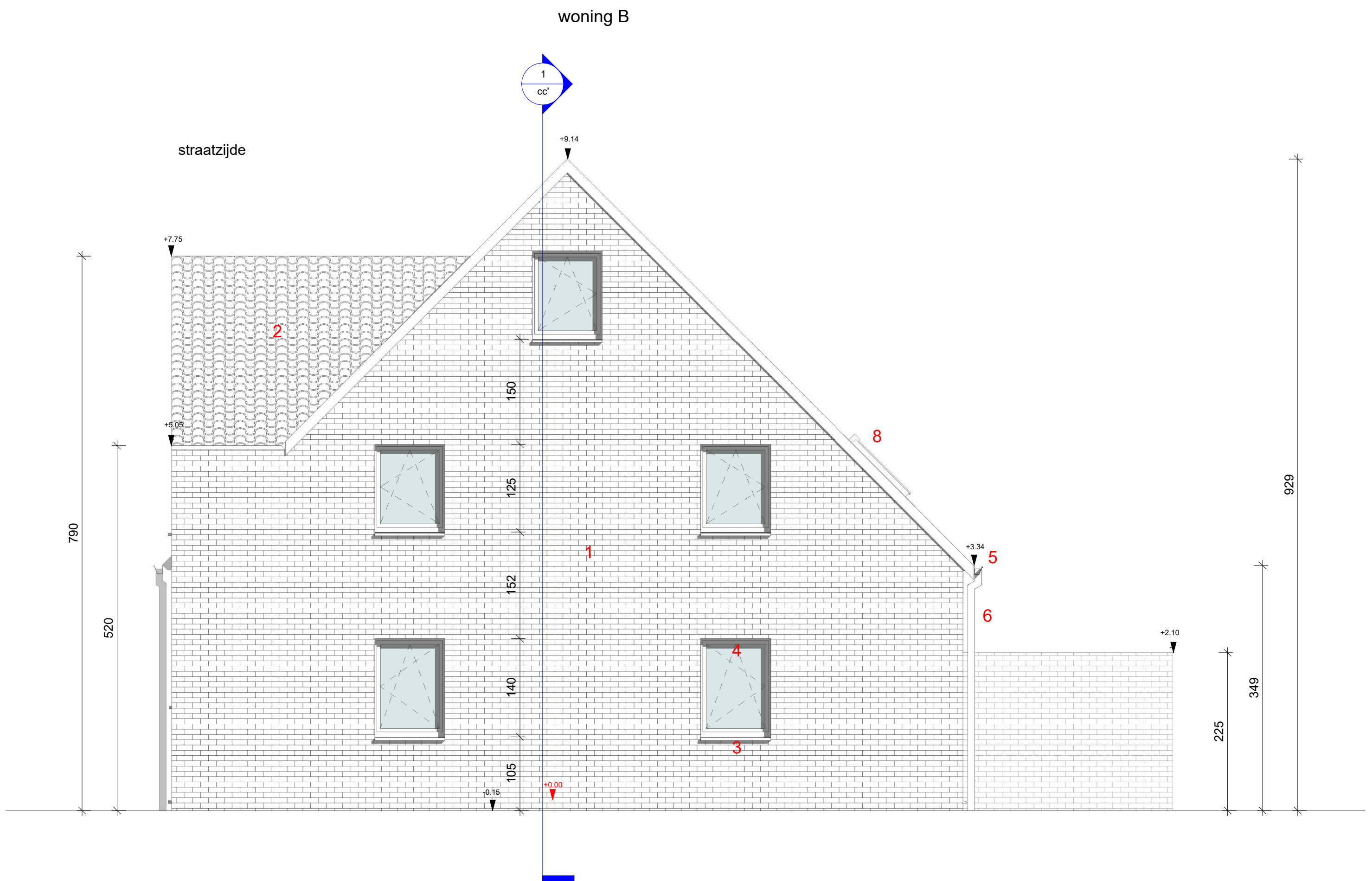
1 BA_woning B_G_N_2_rechterevel 1 : 50
