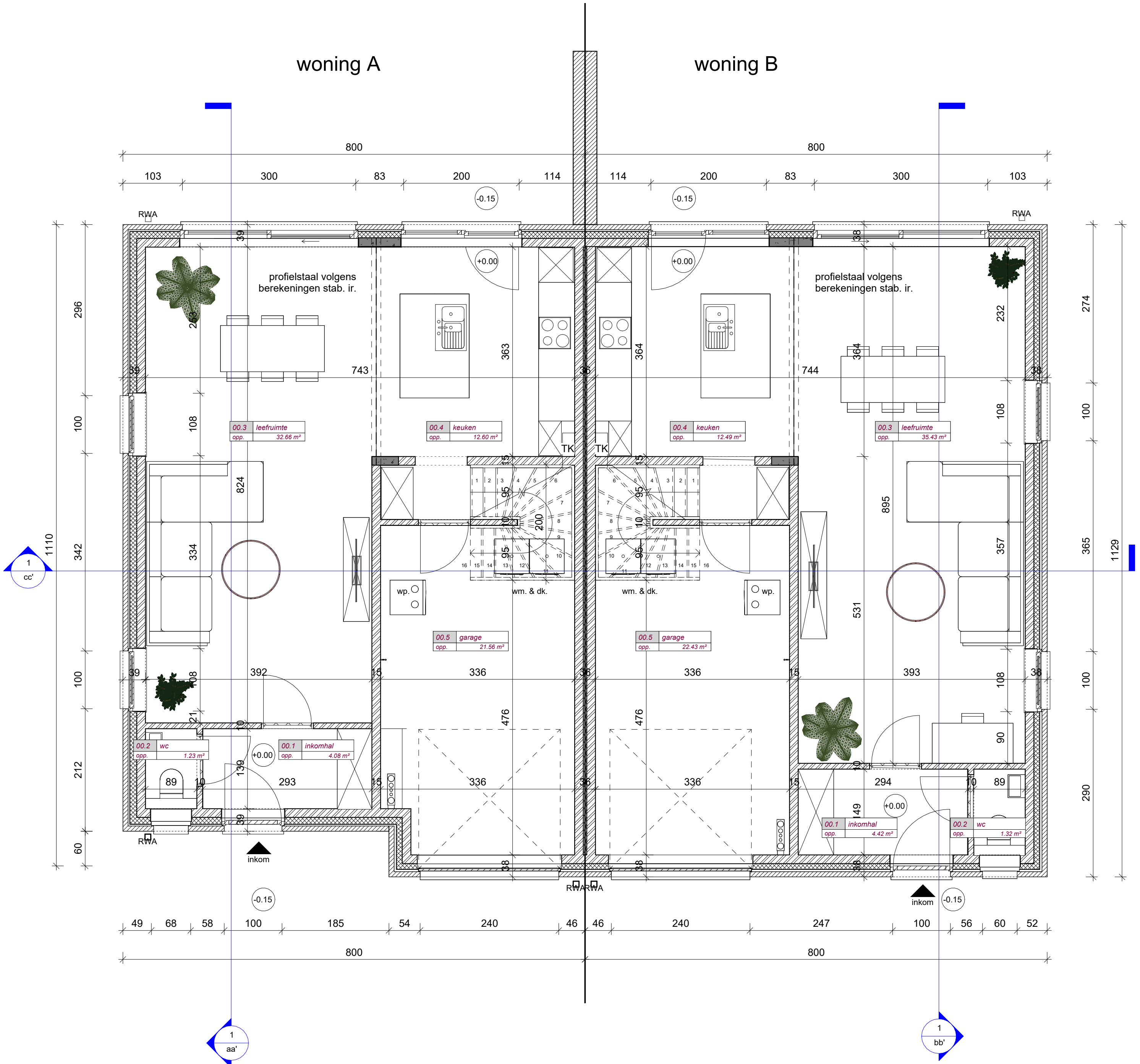
1 BA_woning A&B_P_N_00_geljkvloers 1 : 50
