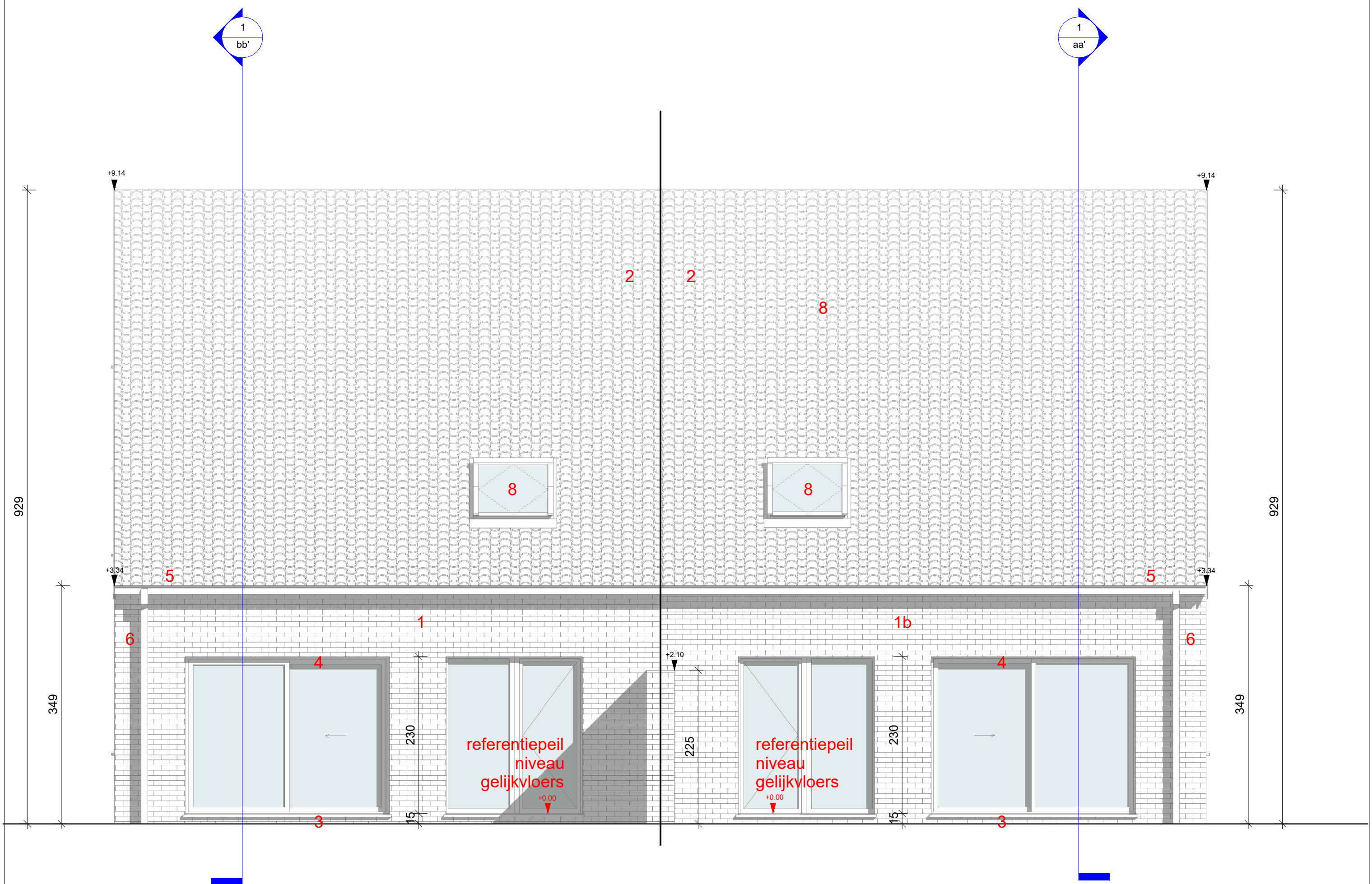
1 BA_woning A&B_G_N_3_achtergevel 1 : 50
