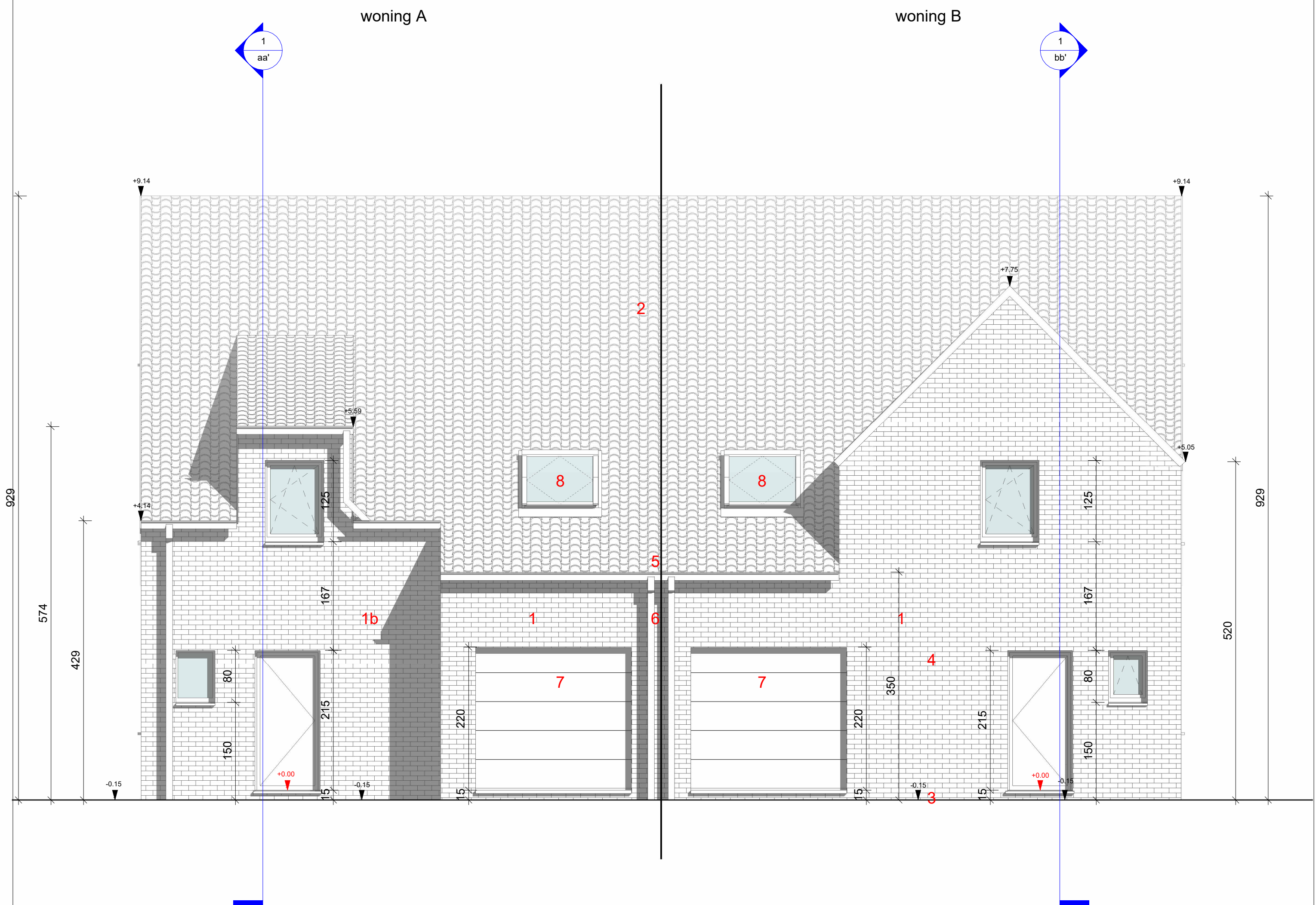
1 BA_woning A&B_G_N_1_voorgevel 1 : 50
